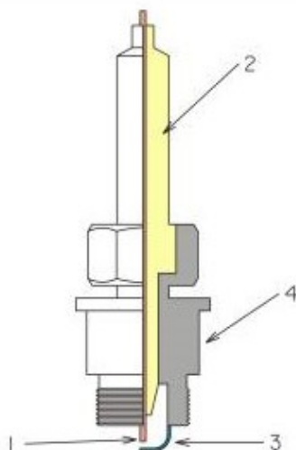
Ilustracja 1: 1 - elektroda centralna, 2 - izolator ceramiczny, 3 - elektroda boczna, 4 - korpus świecy
